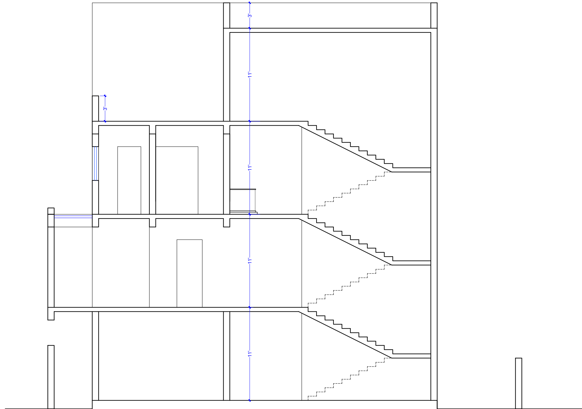
SECTION A-A'
